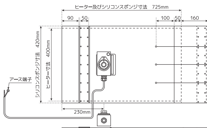
■形状図：47Lボンベ用ヒーター
